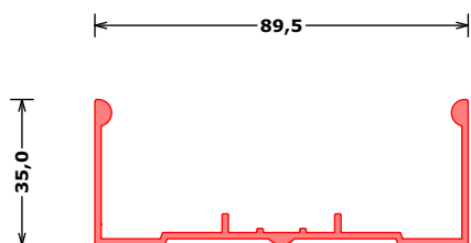
171980*** UP DG-SL vloerprofiel DG vlak | floor track DG flat | Bodenprofil DG flach
