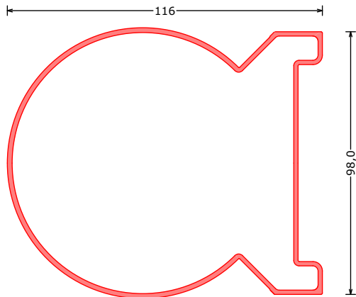
171791*** HPH hoekprofiel rond 90-270° | cover profilr rond 90-270° Eckprofil 90-270° abgerundet L=6200mm
