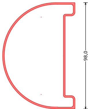
171772*** HP180ST wandbeëdigingsprofiel rond | cornerprofile 180° wandbeëdigungs profil 180° L=6200mm
