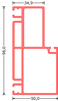
171830*** RDK RECHT 3D deurprofiel recht 3D verstelbaar scharnier doorprofile square for adjustable hinges Türzarge für 3D-Bänder rechtwinklich L=6100mm
