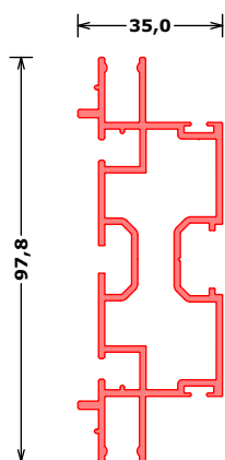
171982*** VV DG-SL verbindingsprofiel DG | connecting profile DG | Verbindungsprofil DG
