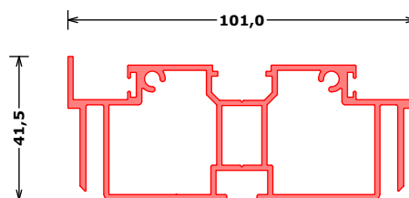
171981*** VP DG-SL vloerprofiel DG verstelbaar | floor track DG adjustable Bodenprofil DG einstellbar
