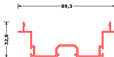
171983*** BPDG DG-SL bovenprofiel DG | upper profile DG | Obenprofil DG
