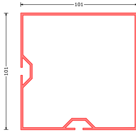
171773*** HPV2 QW98 hoekprofiel 90° recht QW98 | cornerprofile 90° sqaure QW98 Eckprofil 90° Rechtwinklich QW98 L=6200mm
