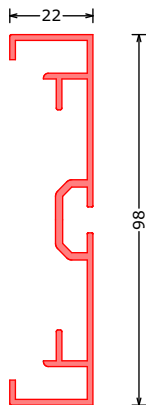
171769*** DS22 QW98 dagstuk 22 QW98 | DS 22 profile QW98 | DS22 profil QW98 L=6100mm
