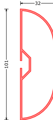
172309*** HP180 QW98 hoekprofiel 180° QW98 | cornerprofile 180° QW98 Eckprofil 180° QW98 L=6100mm
