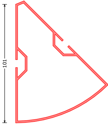
172311*** HP45 QW98 hoekprofiel 45° QW98 | cornerprofile 45° QW98 Eckprofil 45° QW98 L=6100mm
