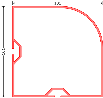
172308*** HP90 QW98 hoekprofiel 90° QW98 | cornerprofile 90° QW98 Eckprofil 90° QW98 L=6100mm
