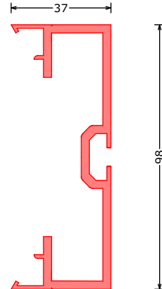
171770*** DS37 QW98 dagstuk 37 QW98 | DS 37 profile QW98 | DS37 profil QW98 L=4400mm
