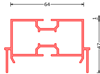
171762*** AP001 UP1 64 CLR verstelbaarprofiel t.b.v. UP1 64 adjustable profile for UP1 64 Einstellbar Profil für UP1 64 L=6100mm
