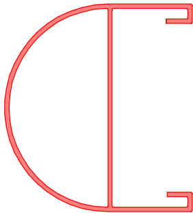
171820*** EPR180S CCS-P80 eindprofiel rond 180° P80 | End profile round 180° P80 Ende Profil abgerundet 180° P80 L=6000mm
