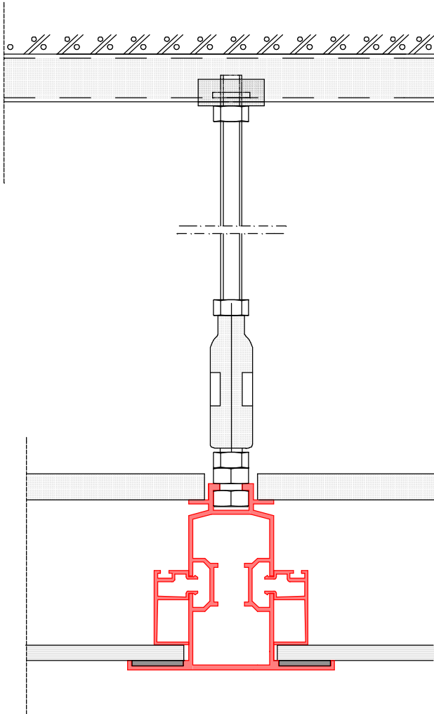
detail A (beloopbaar)
