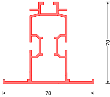
171758*** CPC CCS-C80 plafondprofiel gesloten 78mm PS78DFC L=6000mm
