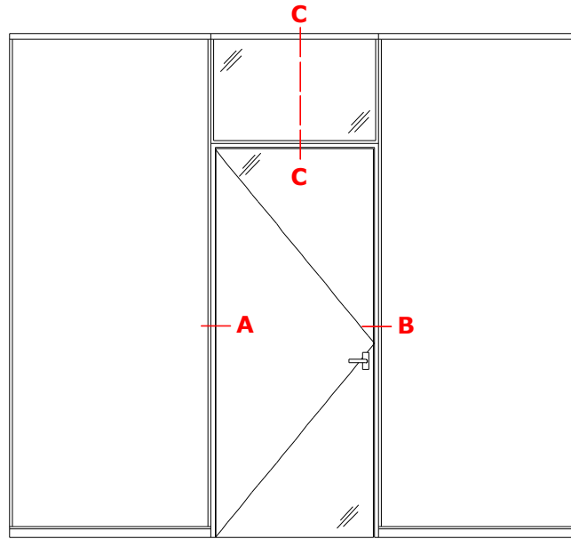
TecnoLine : moduul DFF-HG
