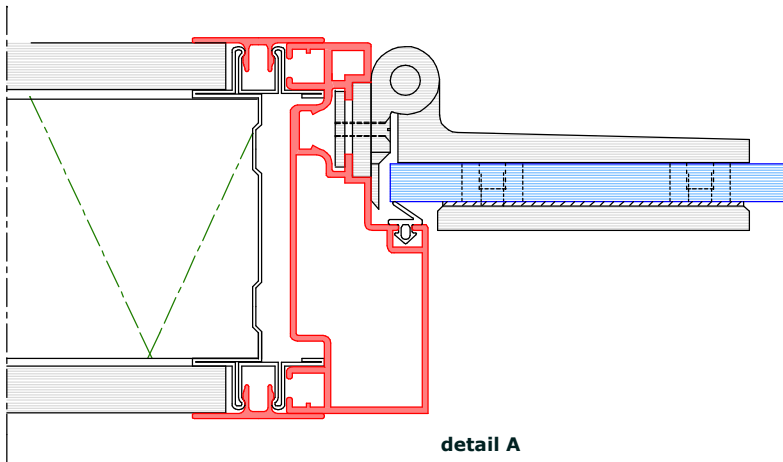
TecnoLine : moduul DDAW-HG
