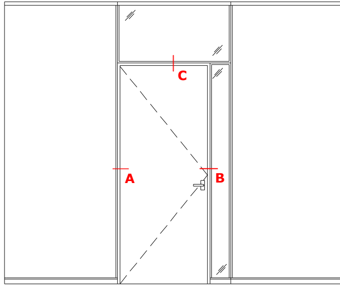
TecnoLine : moduul DBB
