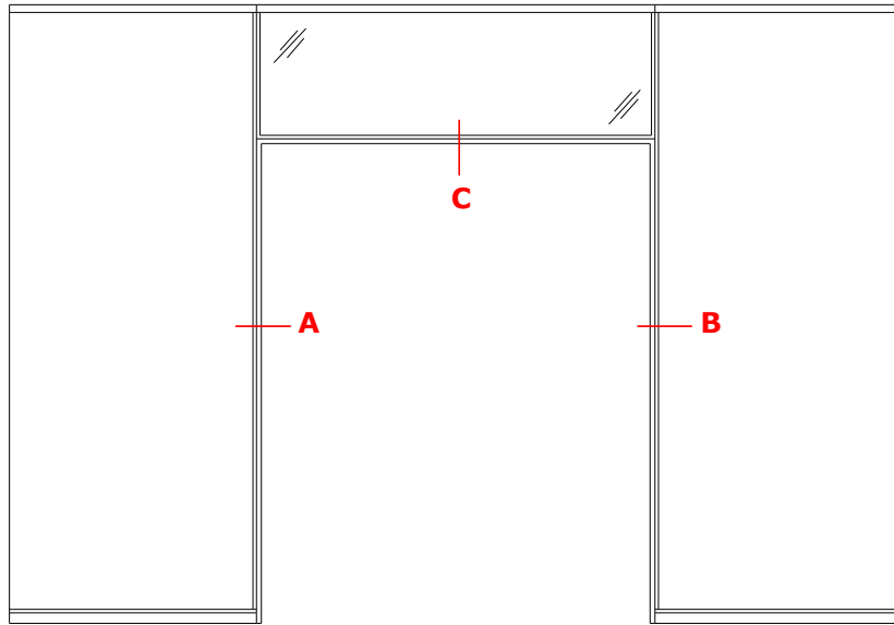
TecnoLine : moduul DDH-DL
