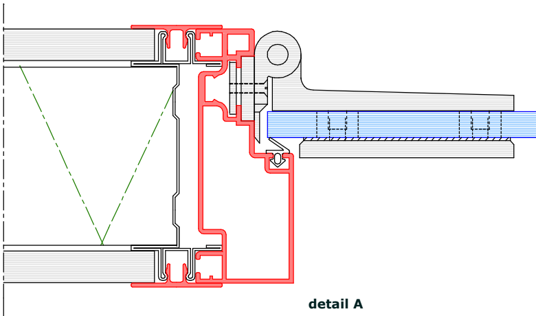
TecnoLine : moduul DDH-HG
