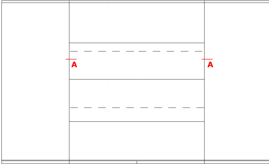
TecnoLine moduul AA4 h.o.h. 2400mm (horizontaal)
