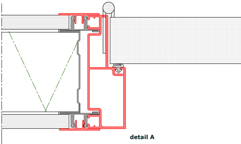
TecnoLine : moduul DDAW
