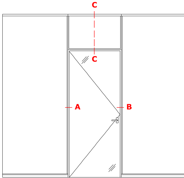
TecnoLine : moduul DGG-HG
