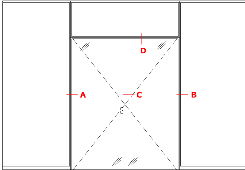
TecnoLine : moduul DME-HG
