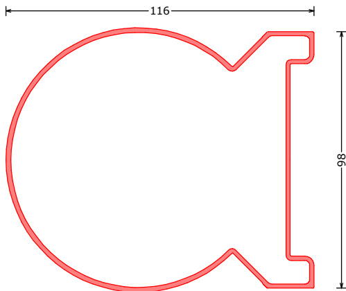
171791*** HPH hoekprofiel rond 90-270° | cover profiel rond 90-270° Eckprofil 90-270° abgerundet L=6200mm
