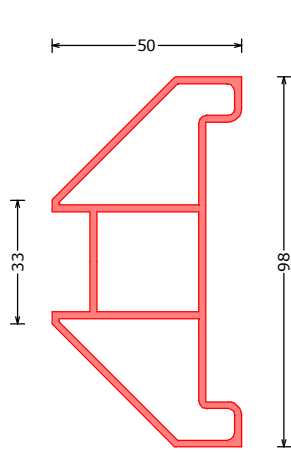
172041*** VJP33/98 verjongingsprofiel 33/98 | narrow profile 33/98 | Verjungsprofil 33/98 L=6100mm
