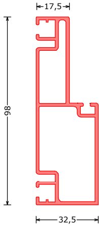
171798*** RDK RECHT deurprofiel recht | doorprofile square | Türzarge rechteckig L=6100mm
