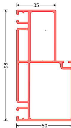
171830*** RDK RECHT 3D deurprofiel recht 3D verstelbaar scharnier doorprofile square for adjustable hinges Türzarge für 3D-Bänder rechtwinklich L=6100mm
