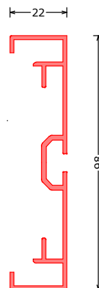
171769*** DS22 QW98 dagstuk 22 QW98 | DS 22 profile QW98 | DS22 profil QW98 L=6100mm
