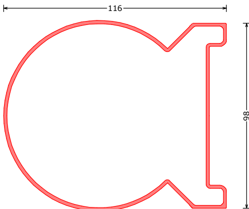
171791*** HPH hoekprofiel rond 90-270° | cover profil round 90-270° Eckprofil 90-270° abgerundet L=6200mm
