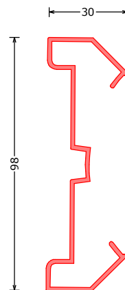
171792*** HPA aansluitprofiel voor HPH | connection profile for HPH Anschlussprofil für HPH L=6200mm
