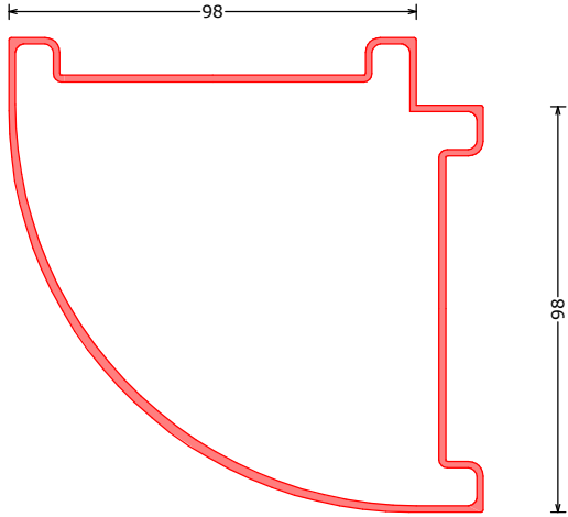
171771*** HP90ST hoekprofiel rond 90° | cornerprofile 90° | Eckprofil 90° abgerundet L=6200mm
