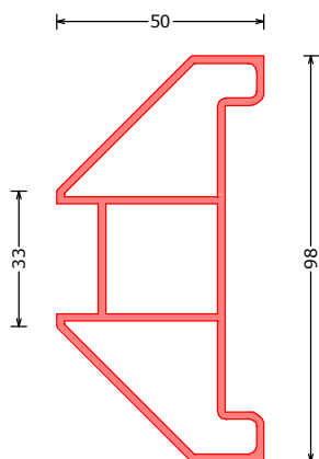
172041*** VJP33/98 verjongingsprofiel 33/98 | narrow profile 33/98 | Verjongingsprofiel 33/98 L=6100mm
