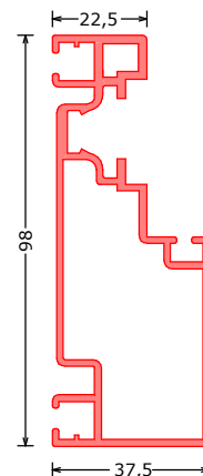
172145*** RDK 15 RECHT deurprofiel recht voor hardglazen deur doorprofile square for glass door Türzarge rechtwinklich für vollglastür L=6100mm
