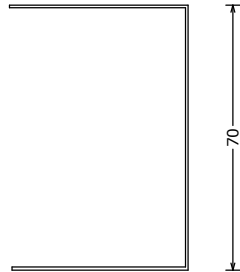
27310000 SM-CST 250 schuifmof CST t.b.v. C50 extension CST for C50 Schiebeteil CST für C50 L=250mm
