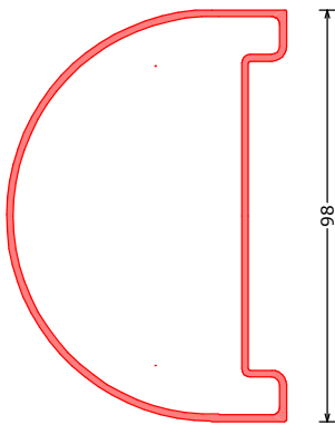
171772*** HP180ST wandbeëidigingsprofiel rond | cornerprofile 180° wandbeëidigungsprofil 180° L=6200mm
