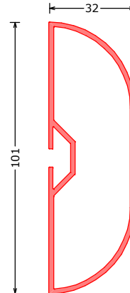
172309*** H180 QW98 hoekprofiel 180° QW98 | cornerprofile 180° QW98 Eckprofil 180° QW98 L=6100mm
