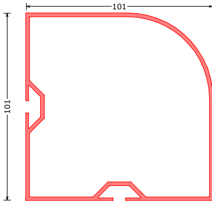
172308*** H90 QW98 hoekprofiel 90° QW98 | cornerprofile 90° QW98 Eckprofil 90° QW98 L=6100mm
