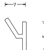
273075000 DR DPS QW deurrubber t.b.v. DPS profiel QW Doorstop gasket for DPS profile Türgummi für DPS Profil
