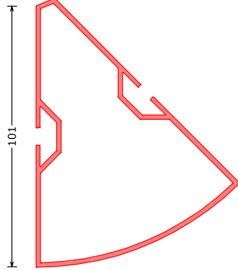
172311*** H45 QW98 hoekprofiel 45° QW98 | cornerprofile 45° QW98 Eckprofil 45° QW98 L=6100mm
