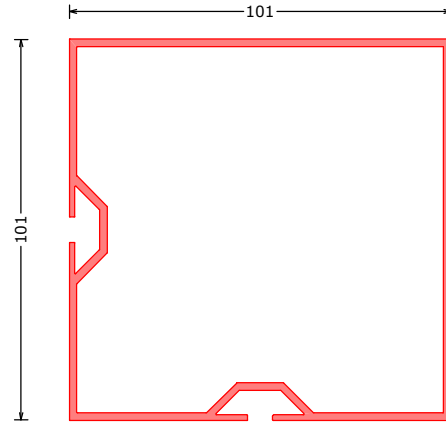
171773*** HPV2 QW98 hoekprofiel 90° recht QW98 | cornerprofile 90° square QW98 Eckprofil 90° Rechtwinklich QW98 L=6200mm
