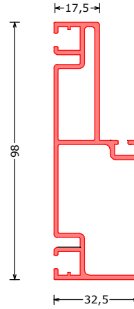
171798*** RDK RECHT deurprofiel recht | doorprofile square | Tüorzarge rechtwinklich L=6100mm
