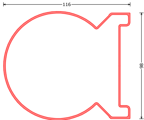
171791*** HPH hoekprofiel rond 90-270° | cover profilr round 90-270° Eckprofil 90-270° abgerundet L=6200mm
