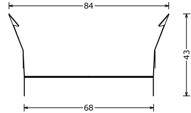
273102000 PB-BP FR plaatbeugel staal FR t.b.v. BP FR Steel Strip FR for BP FR Plattenbügel für BP FR L=50mm
