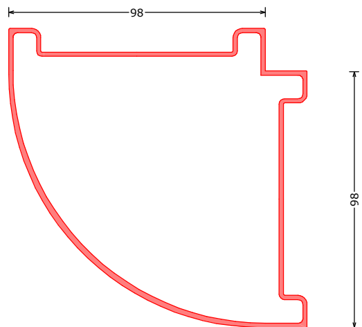
171771*** HP90ST hoekprofiel rond 90° | cornerprofile 90° | Eckprofil 90° abgerundet L=6200mm
