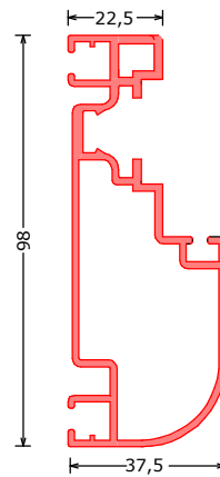
171796*** RDK 15 deurprofiel rond voor hardglazen deur doorprofile round for glass door Tüorzarge abgerundet für vollglastür L=6100mm
