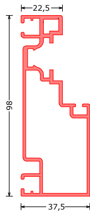
172145*** RDK 15 RECHT deurprofiel recht voor hardglazen deur doorprofile square for glass door Tüorzarge rechtwinklich für vollglastür L=6100mm
