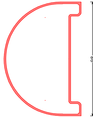
171772*** HP180ST wandbeëdigingsprofiel rond | cornerprofile 180° wandbeeindigungsprofil 180° L=6200mm
