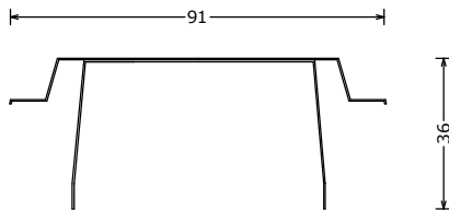
273032000 PB-VP FR plaatbeugel staal FR t.b.v. VP Steel Strip FR for VP Plattenbügel für VP L=50mm
