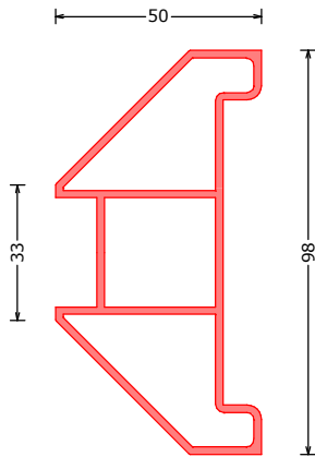
172041*** VJP33/98 verjongingsprofiel 33/98 | narrow profile 33/98 | Verjungsprofil 33/98 L=6100mm
