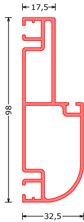
171797*** RDK deurprofiel rond | doorprofile round | Tüorzarge abgerundet L=6100mm
