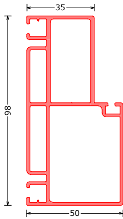
171830*** RDK RECHT 3D deurprofiel recht 3D verstelbaar scharnier doorprofile square for adjustable hinges Tüorzarge für 3D-Bänder rechtwinklich L=6100mm
