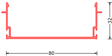
171793*** BPDG bovenprofiel dubbelglas | upper profile double glass | Doppelverglasung für BP L=6100mm
